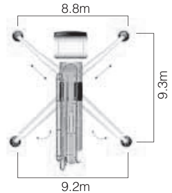
Ausleger
